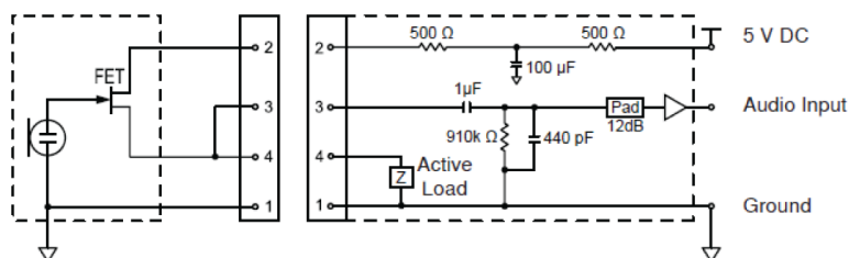
TA4M Connector
