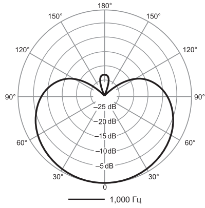
Диаграмма направленности
