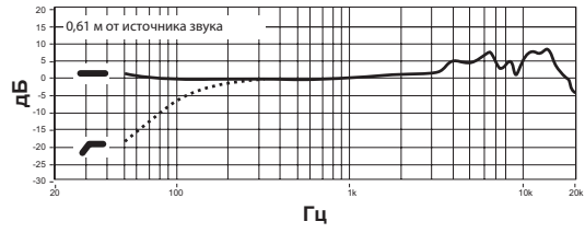
Частотная характеристика
