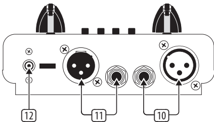
Рис. 2.2: Задняя панель MIC200
