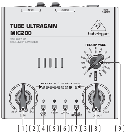
Рис. 2.1: Передняя панель MIC200
